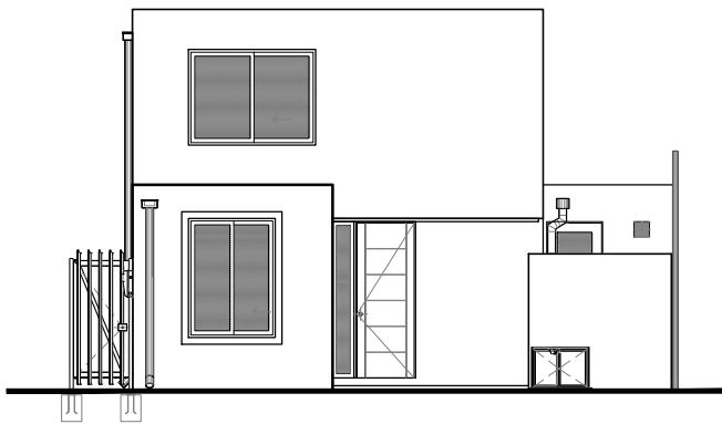
ELEVACION PRINCIPAL
