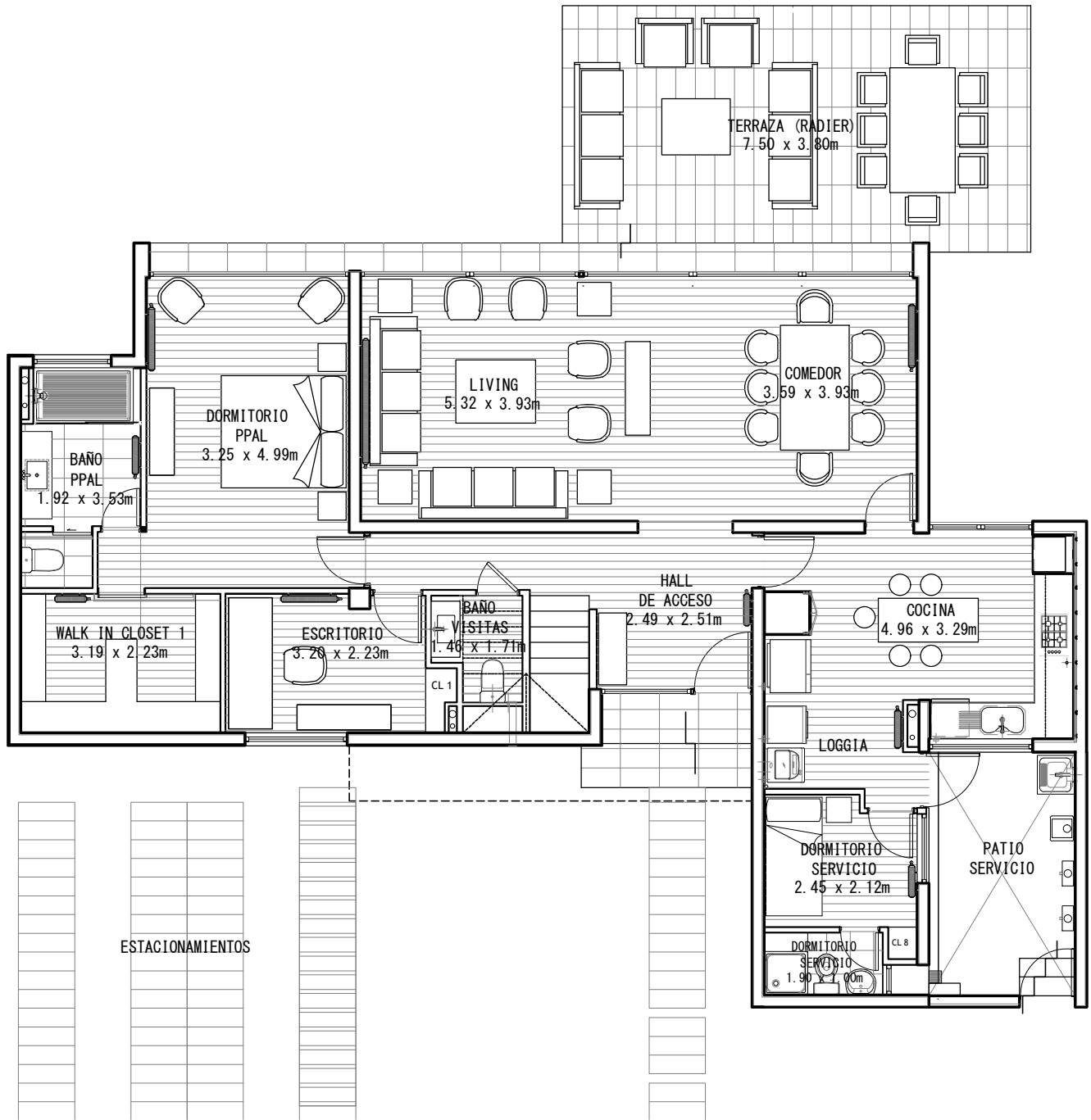
PLANTA PISO 1 PATIO SERVICIO FRONTAL
